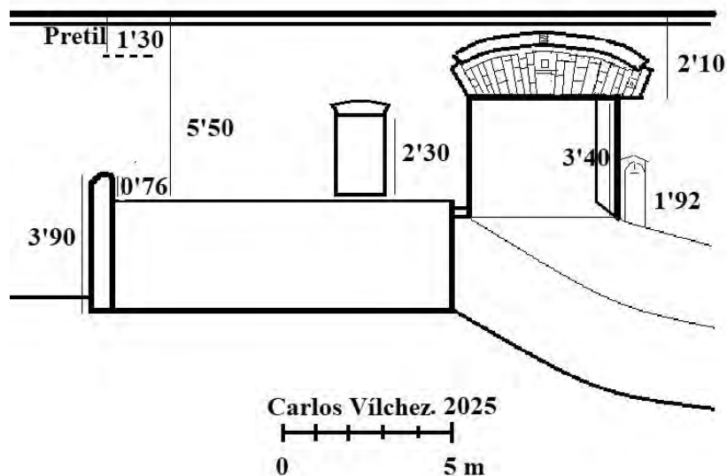
Lámina 13. Alzado de la puerta del Carril o de los Carros. (C. Vilchez, 2025).
